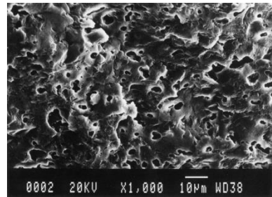
軽量強化磁器の磁器内部の構造 (数 \mu\text{m} の気孔が素地中に多数存在)
