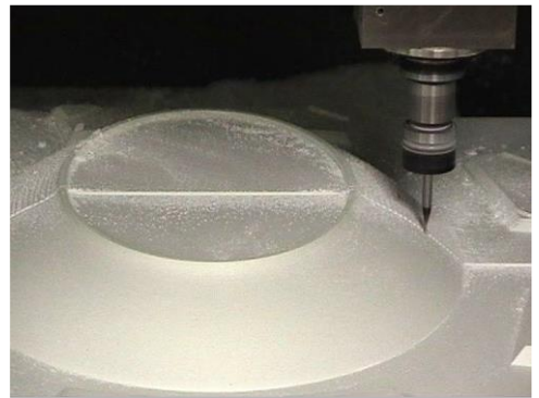
モデリングマシンによる型切削
