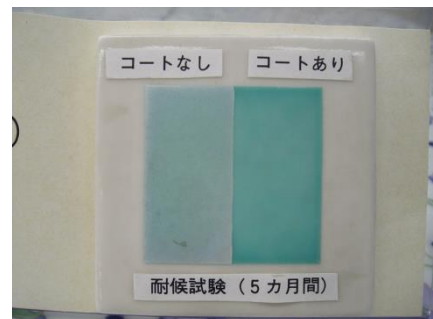
耐候試験結果(酸性雨対策)
