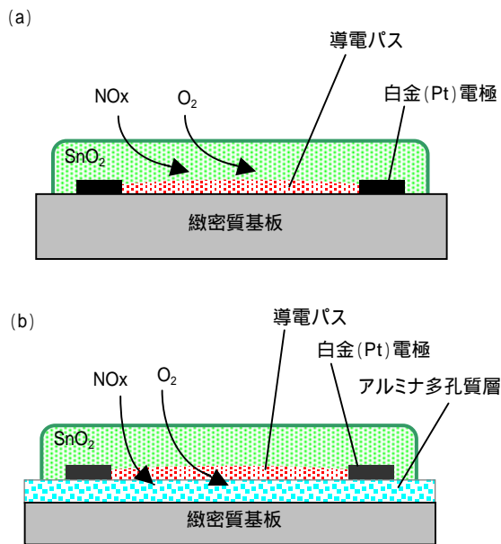
図6 センサ素子におけるガス透過の違い(a)緻密質基板 (b)多孔質基板
