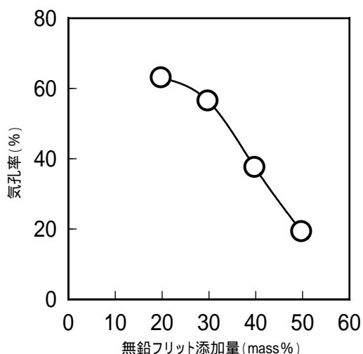
図2 無鉛フリットの添加量に対するアルミナ層(800℃焼成)の気孔率変化
