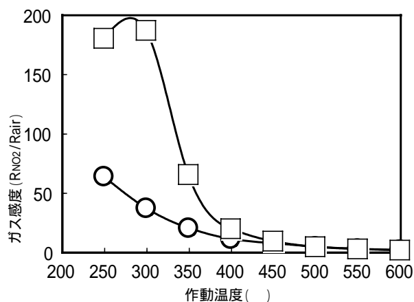
図5 SnO 2 厚膜センサの 88ppm NO 2 に対するガス感度 (○:緻密質基板、□:アルミナ多孔質基板)
