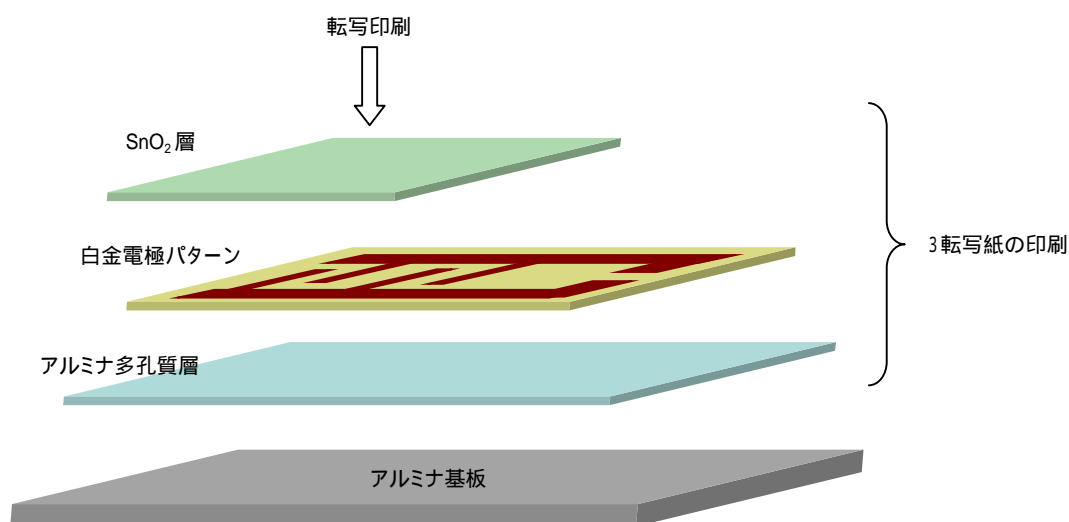
図1 800 °C の1回焼成で得られるセンサ素子の転写紙積層モデル
