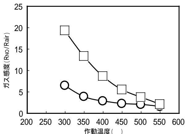
図4 SnO 2 厚膜センサの 771ppm NO に対するガス感度 (○:緻密質基板、□:アルミナ多孔質基板)
