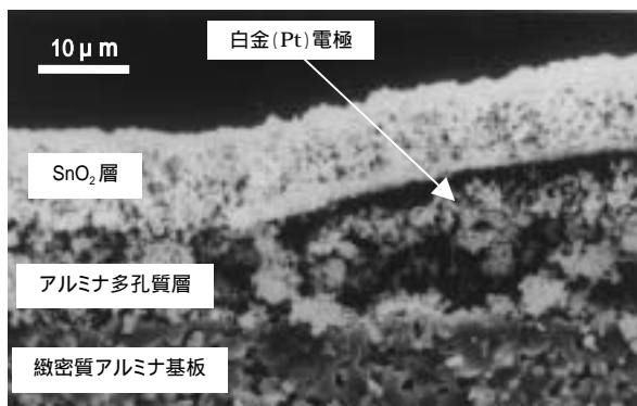
図3 アルミナ多孔質層を用いたセンサ素子断面図(800℃×2hr焼成)
